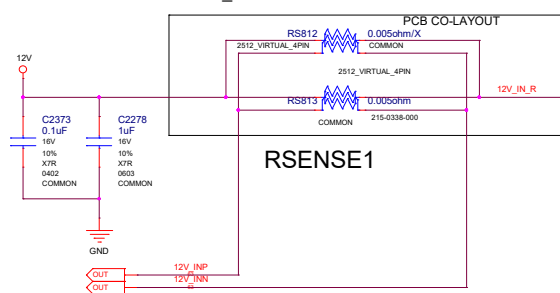
PEX_12V INPUT - 66W
